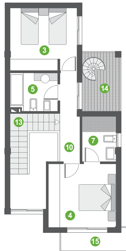
Planta 1ª / First floor
